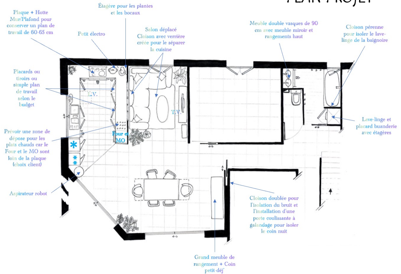
PLAN PROJET
